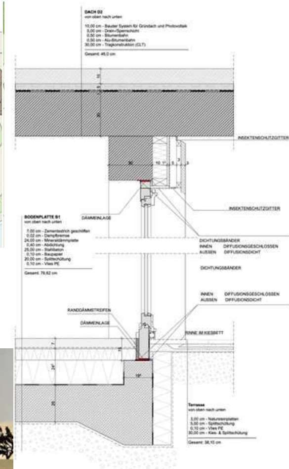
Fassadenschnitt Fenster Pavillon
